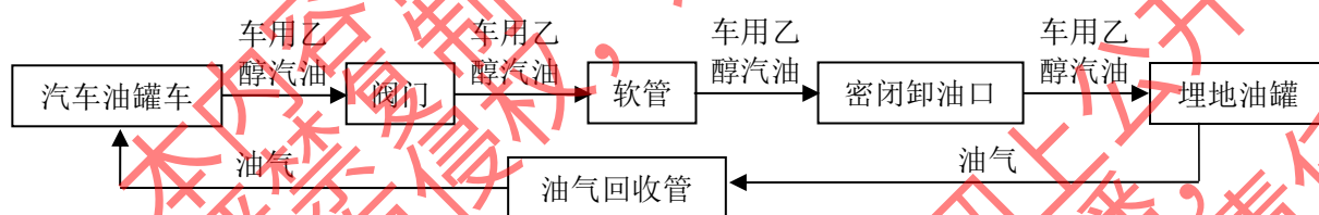
汽油卸油工艺流程图
